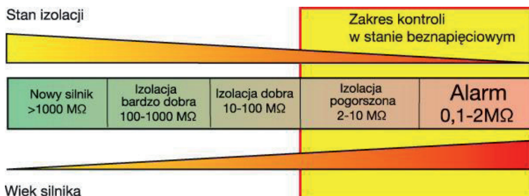
Rys. 1. Przebieg wartości rezystancji silnika w czasie.
