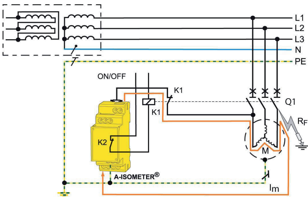
Rys. nr 2. Idea kontroli off- line stanu izolacji silników niskiego napięcia (do ok. 790V)
