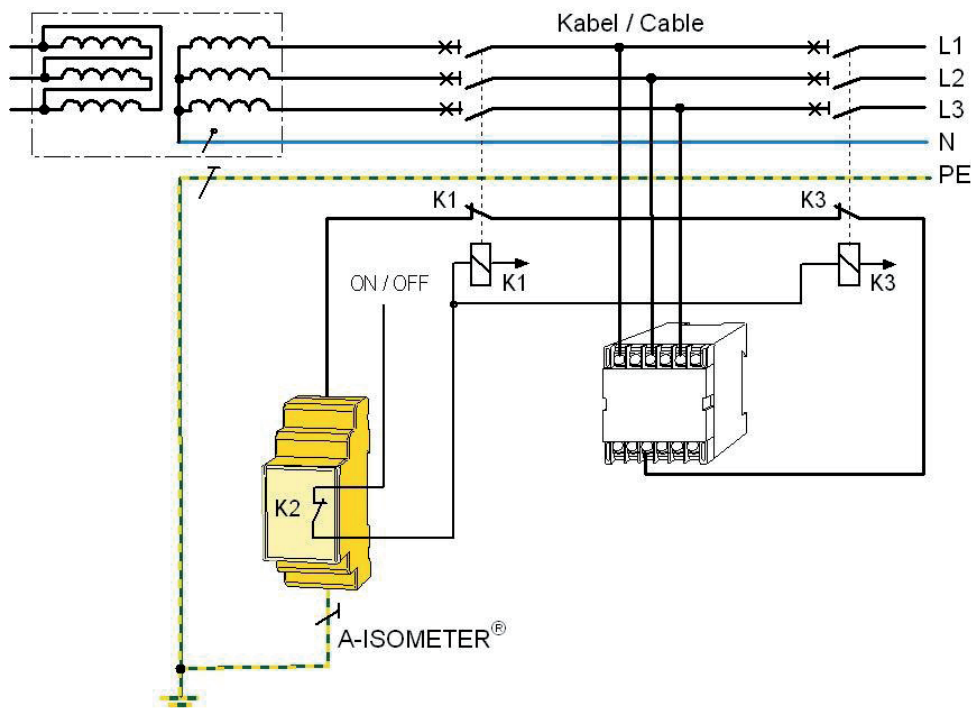
Rys. nr 4. Kontrola off-line stanu izolacji kabli odłączonych od napięcia.
