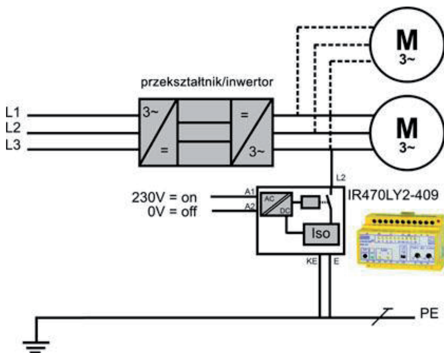
Rys. nr 5. Kontrola off-line izolacji napędów regulowanych.
