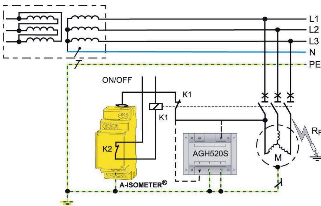
Rys. nr 3. Monitoring off-line silników 6kV.
